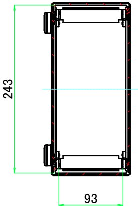
B-B ( 1 : 5.5 )
